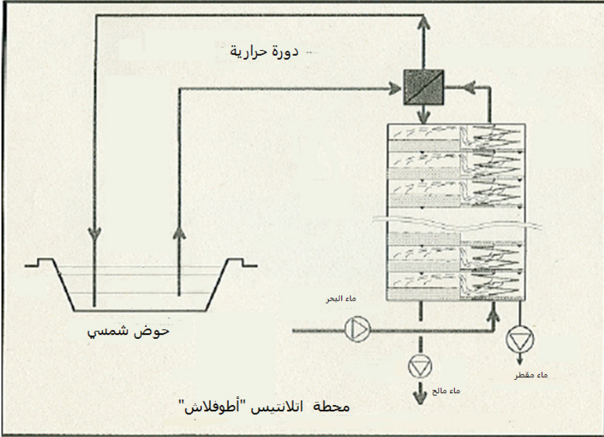
الشكل 14 : الرسم البياني لمحطة التحلية اتلانتيس باستخدام البركة الشمسية المقترنة بالتبخير فلاش [44]
