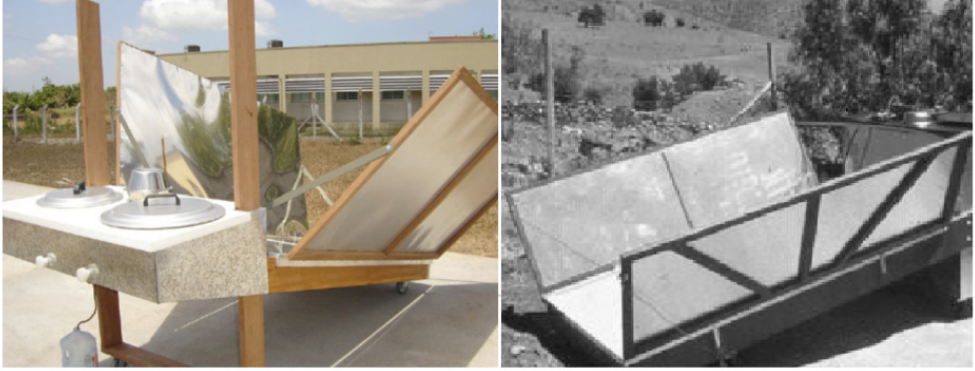
الشكل 16: الطباخات الشمسية غير المباشرة مع مجمع شمسي مسطح في تشيلي (1) وفي البرازيل (2)
