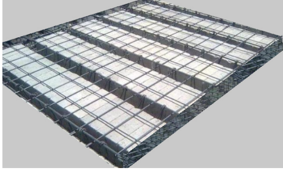
الشكل 8: صورة لبلاطة مفرغة
