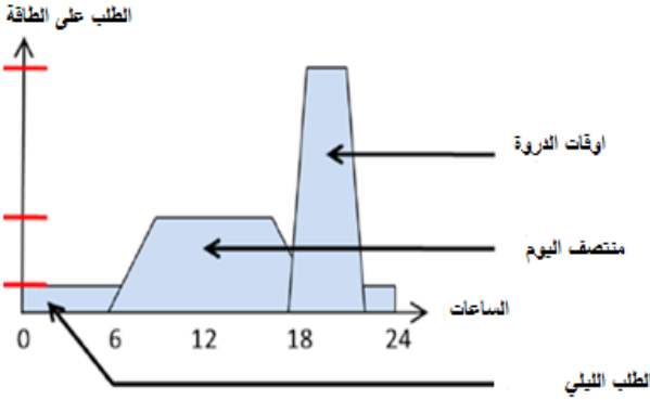
الشكل 3 : منحني الطلب على الطاقة النموذجي في المناطق الريفية [7].
