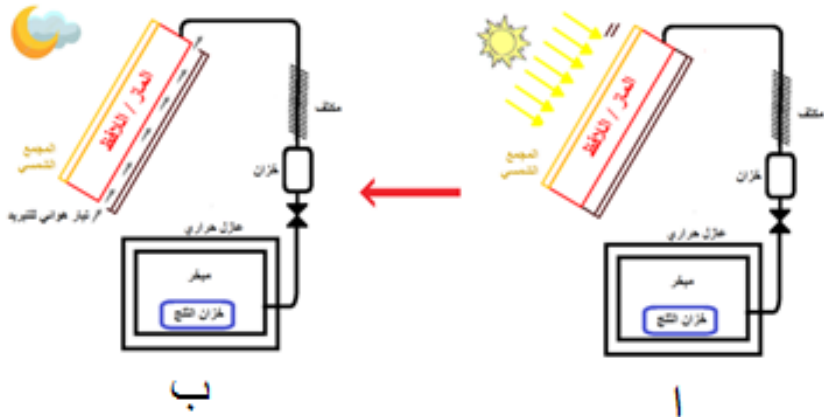
الشكل 15: آلة التبريد الشمسي بالامتزاز التي تعمل وفقا لدورة التأثير المفرد
