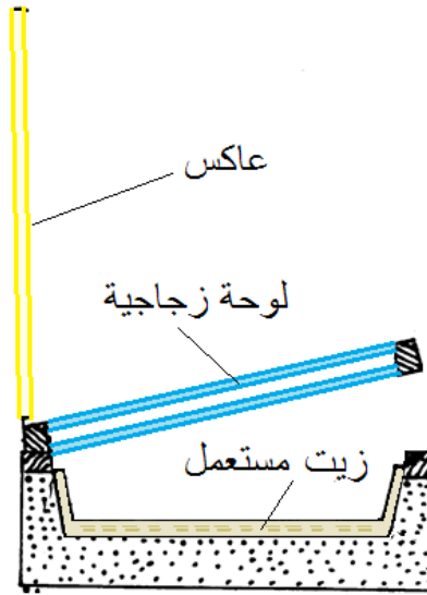
الشكل 18 : صندوق الطهي مع نظام بسيط لتخزين الحرارة المحسوسة
